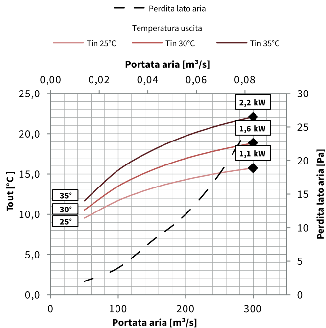
Batteria REO DEH 300 (+7°C/+12°C)
